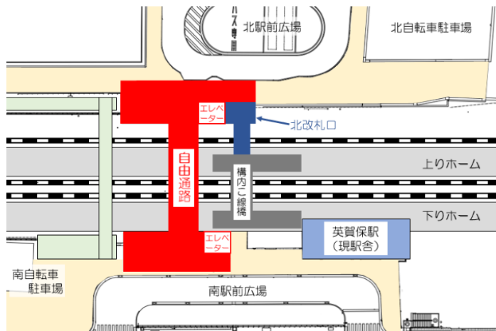
英賀保駅 平面図
