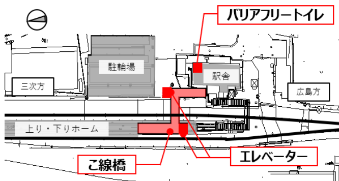
安芸矢口駅構内平面図
