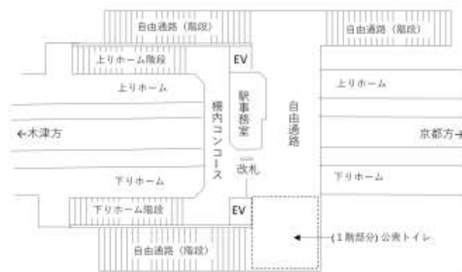
橋上駅・自由通路 平面図
