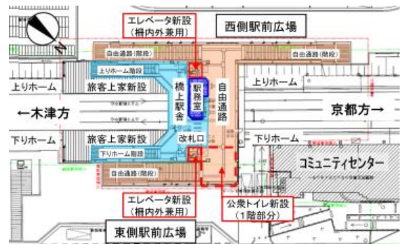
橋上駅・自由通路 平面図
