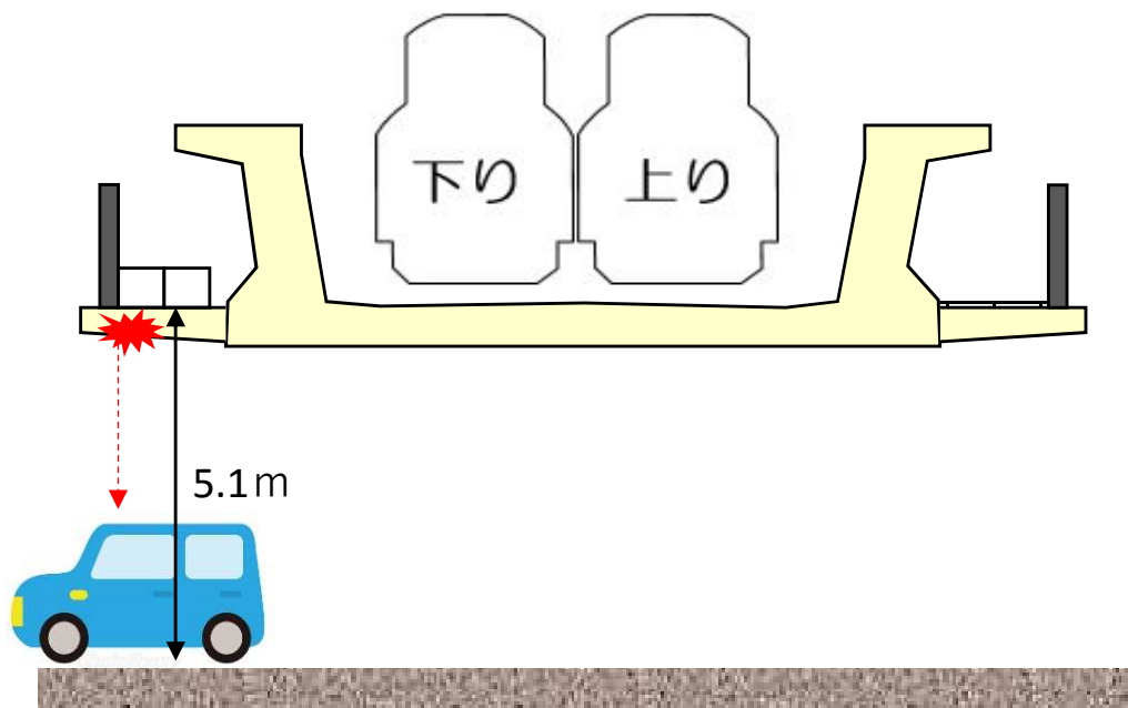
図-1 落下状況断面略図
