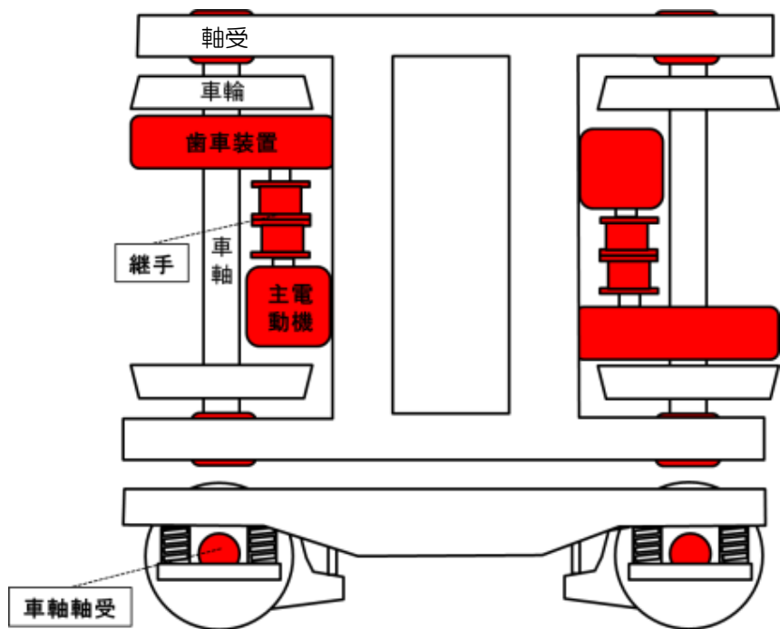
台車故障発生部位
