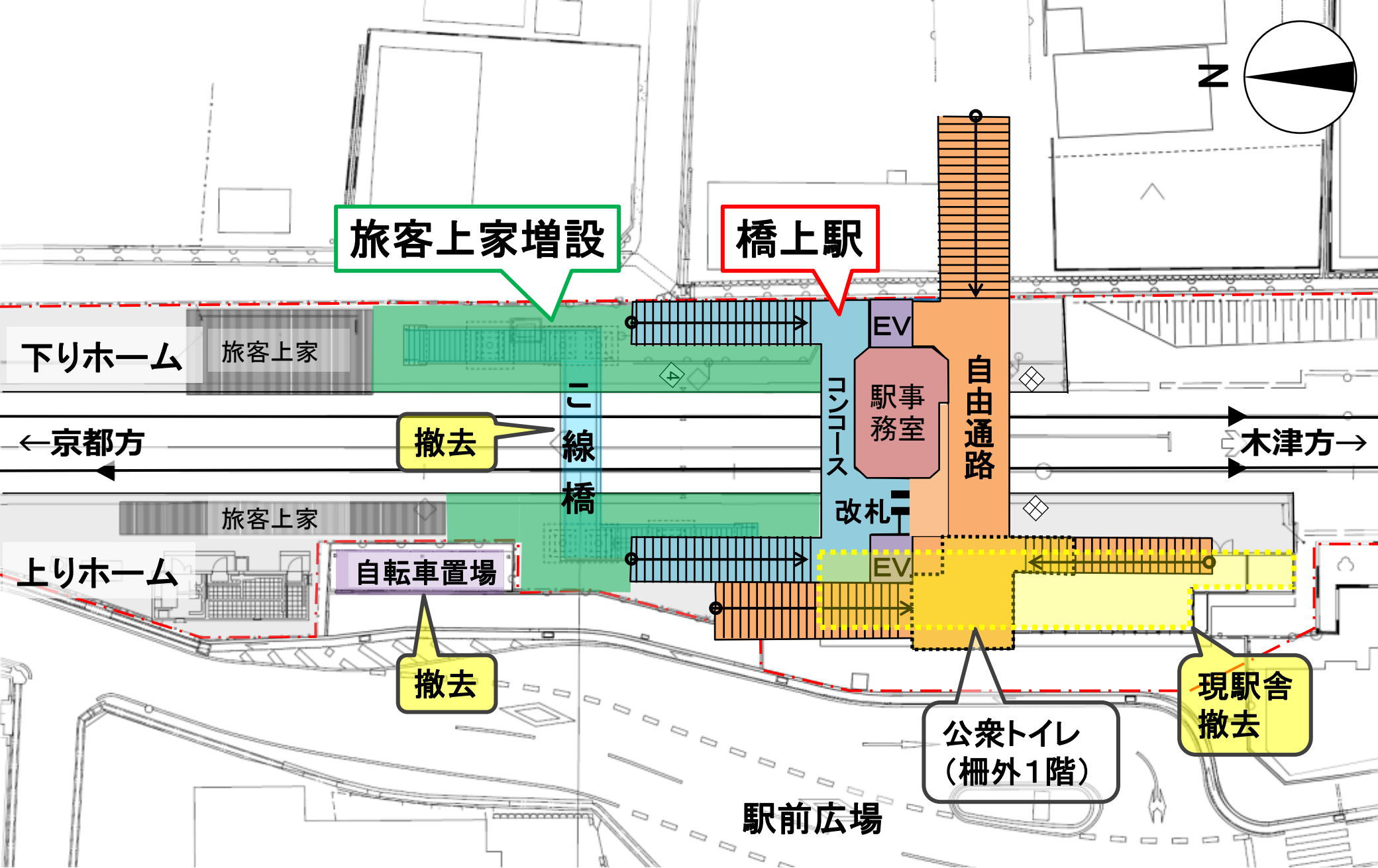
配置図
