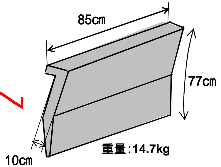
落失・変形した蓄電池箱蓋模式図
