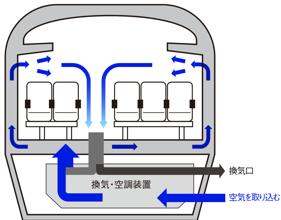
(新幹線車両)
