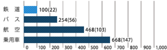
単位輸送量あたりのCO 2 排出量【旅客】（平成25年度）
