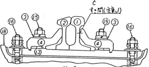
断面 C-C
