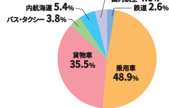
■運輸部門の輸送機関別CO 2 排出量の内訳 (2001年度)
