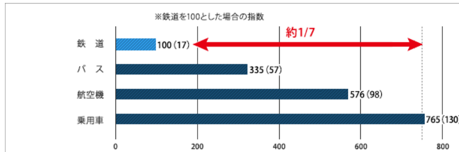
単位輸送量あたりのCO 2 排出量【旅客】（2019年度）
