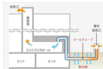
パッシブ換気システム概念図
