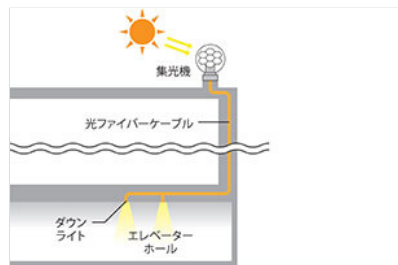
太陽光採光システム概念図
